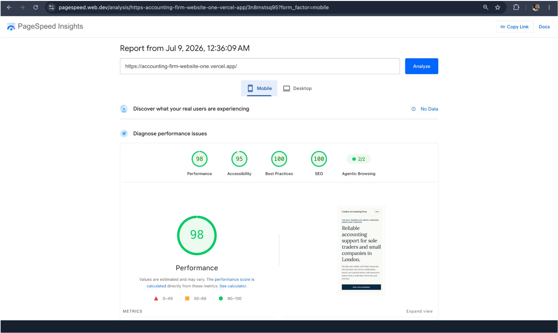
pagespeed-mobile-final.png
